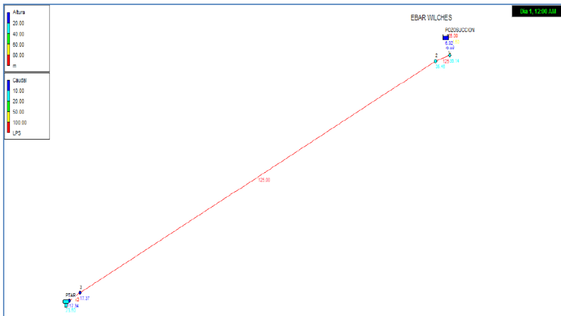
Imagen 5. Modelación de la línea de impulsión elaborada en EPANET.
