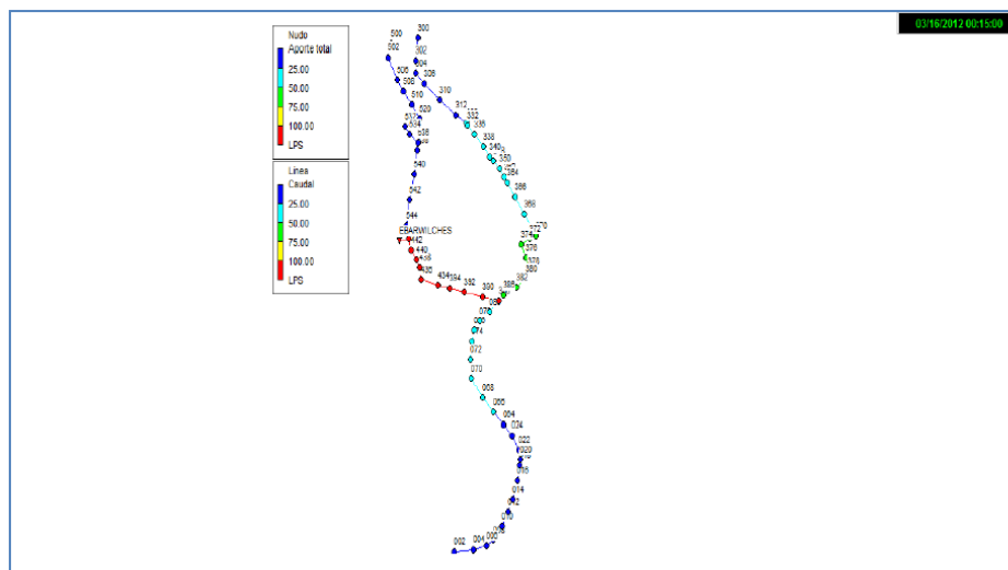
Imagen 4. Dibujo realizado en EPASWMM 5.0 de las redes de alcantarillado sanitario de Wilches.
